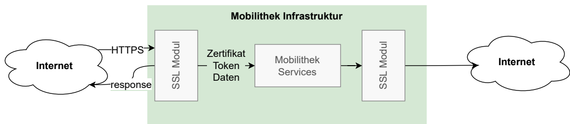
Abbildung 5: Übersicht Sicherheitsarchitektur
